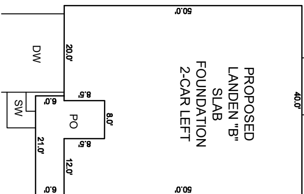
INSET SCALE: 1" = 20'
