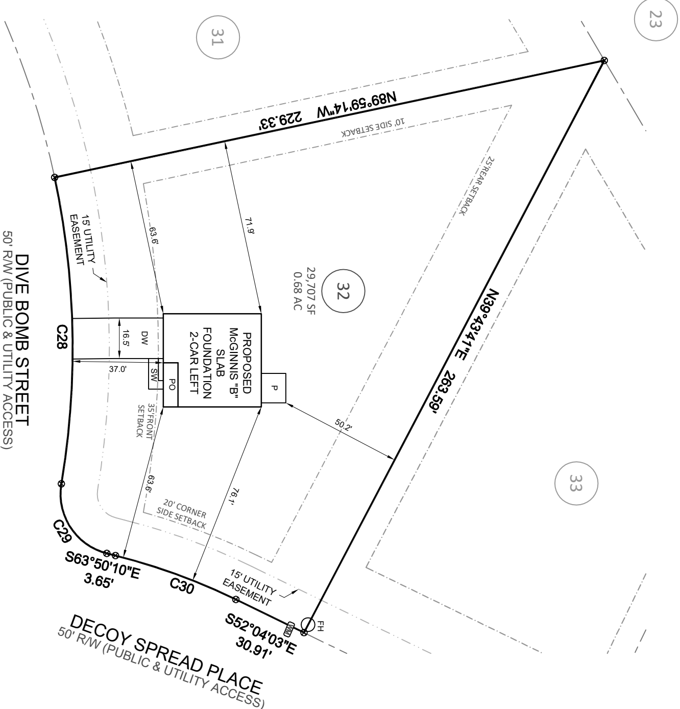
SCALE: 1" = 40 ft.
