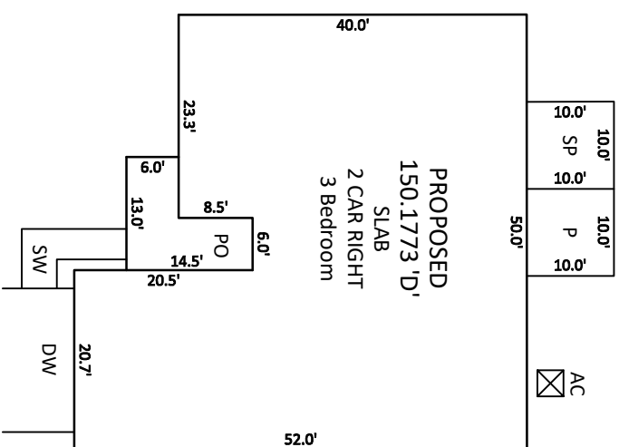
INSET SCALE: 1"=20'
