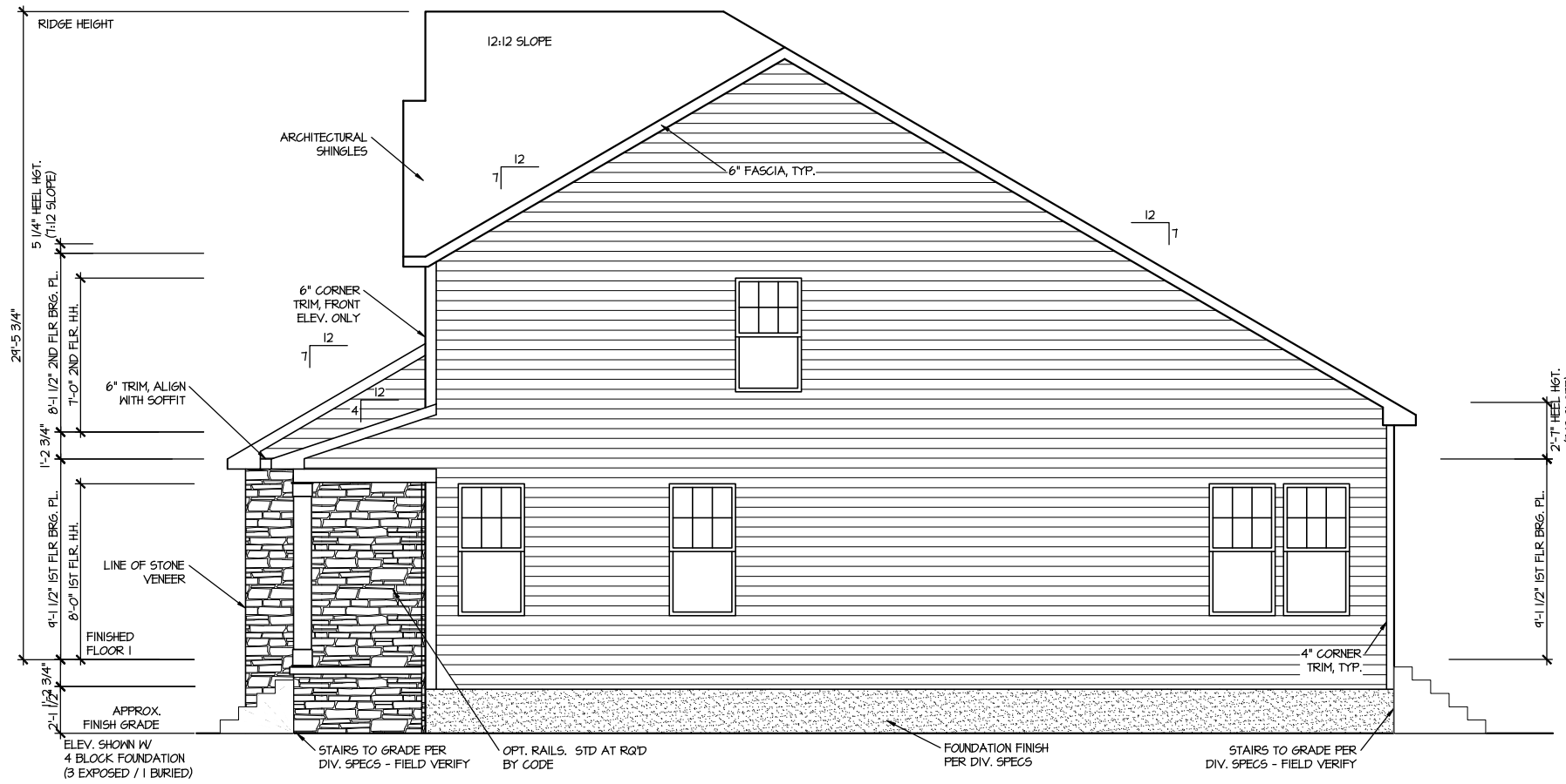
RIGHT ELEVATION 4
