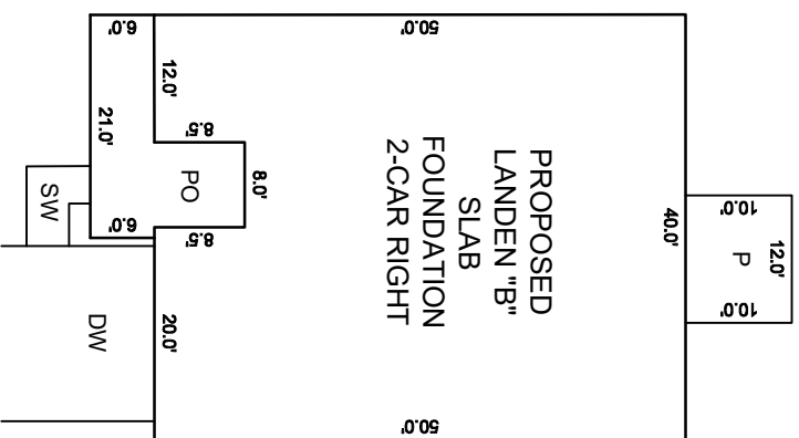
INSET SCALE: 1" = 20'
