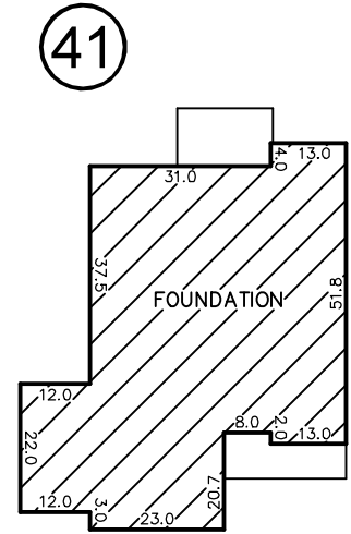
INSET N.T.S.
