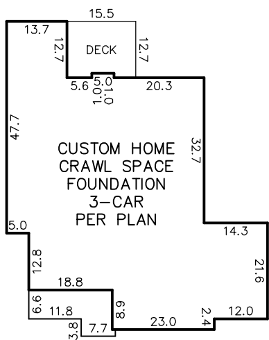
INSET N.T.S.
