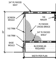
SCALE: 3/4" = 1'-0"
