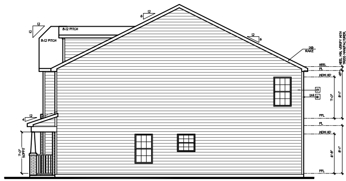
Right Elevation 'B'
