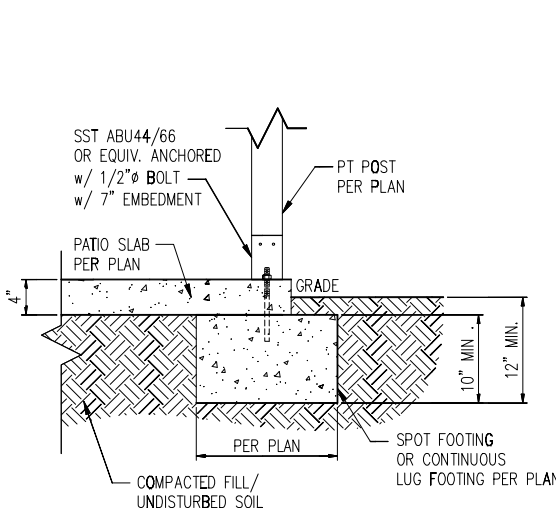
6A COVERED PATIO DETAIL D1m N.T.S.
