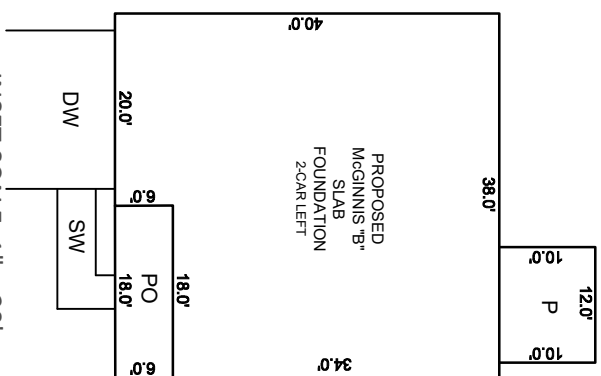
INSET SCALE: 1" = 20'
