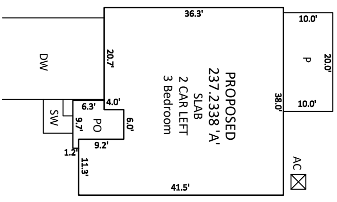
INSET SCALE: 1"=20'
