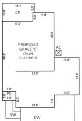
INSET SCALE: 1"=20'
