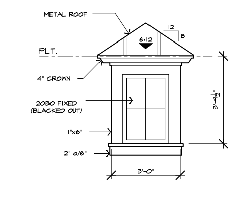
TYP. HIP DORMER
