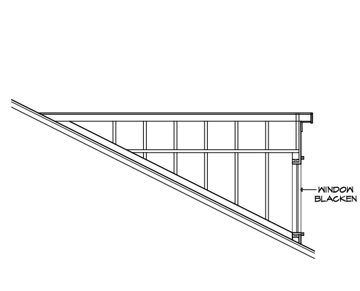
TYP. DORMER
