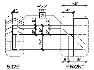
DETAIL 'B' SCALE: N.T.S.
