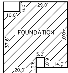
INSET N.T.S.
