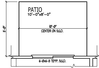
OPT. PATIO
