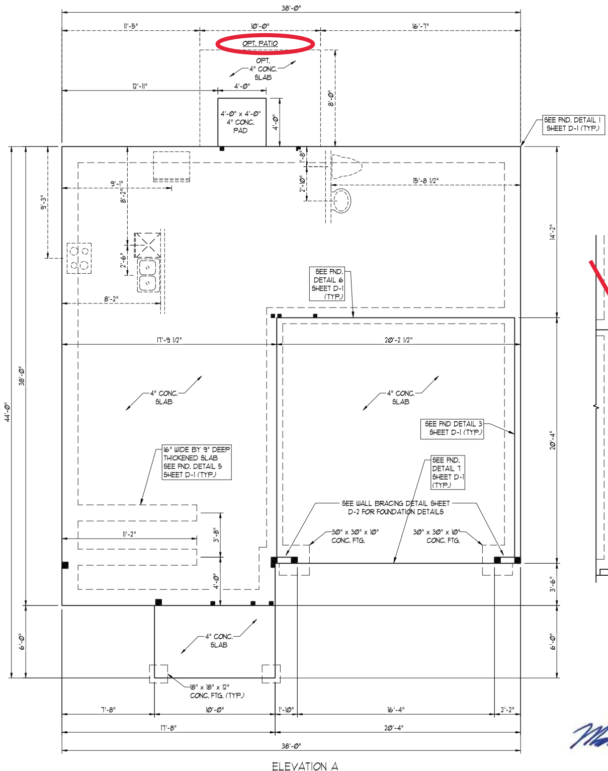
ELEVATION A
