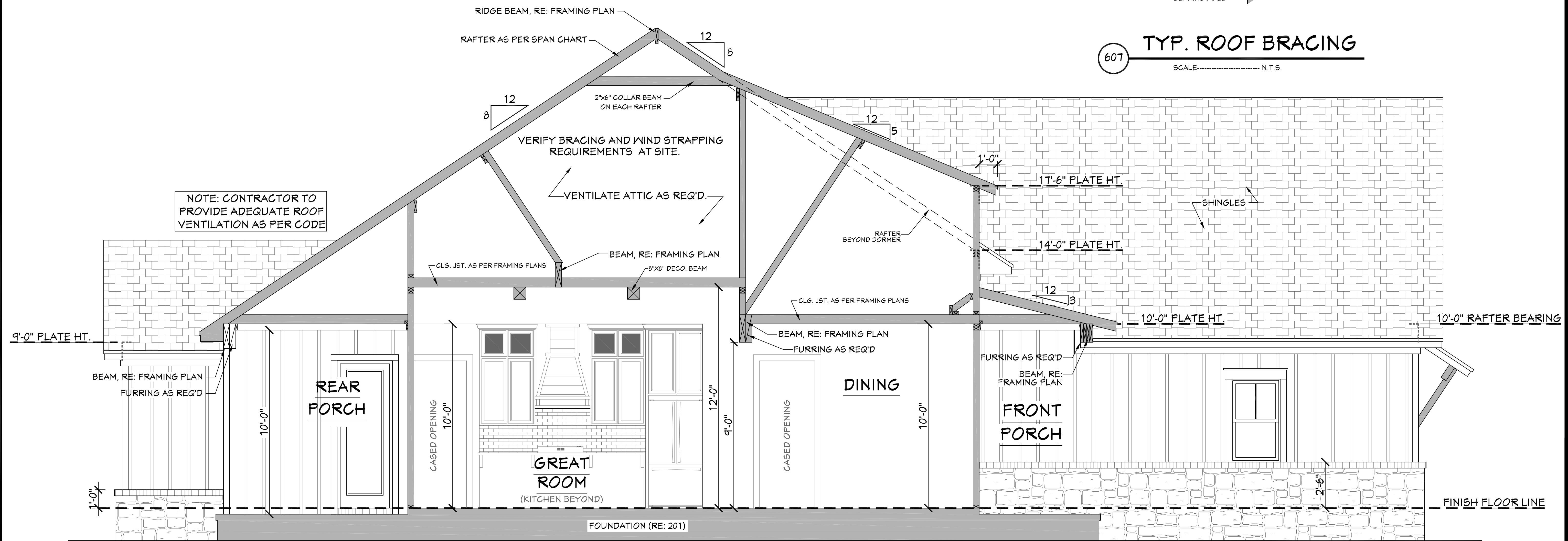
601 CROSS SECTION SCALE: 3/8" = 1'-0"
