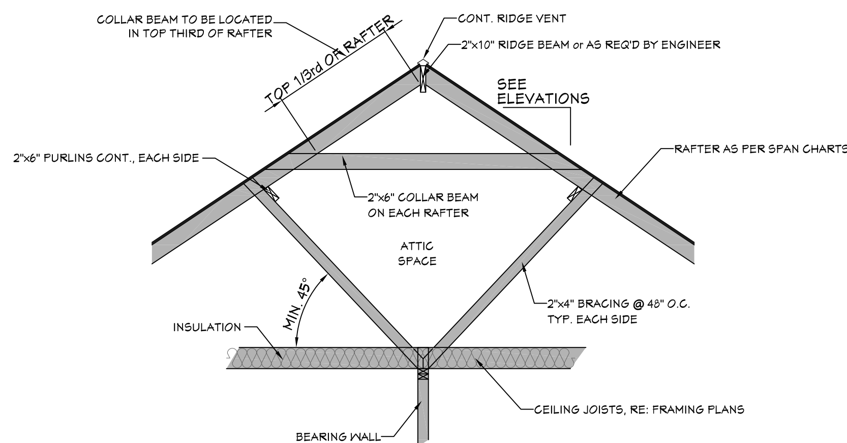
703 TYP. ROOF BRACING SCALE----- N.T.S.
