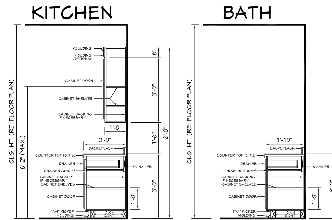
606 TYPICAL CABINET SECTIONS SCALE: N.T.S.
