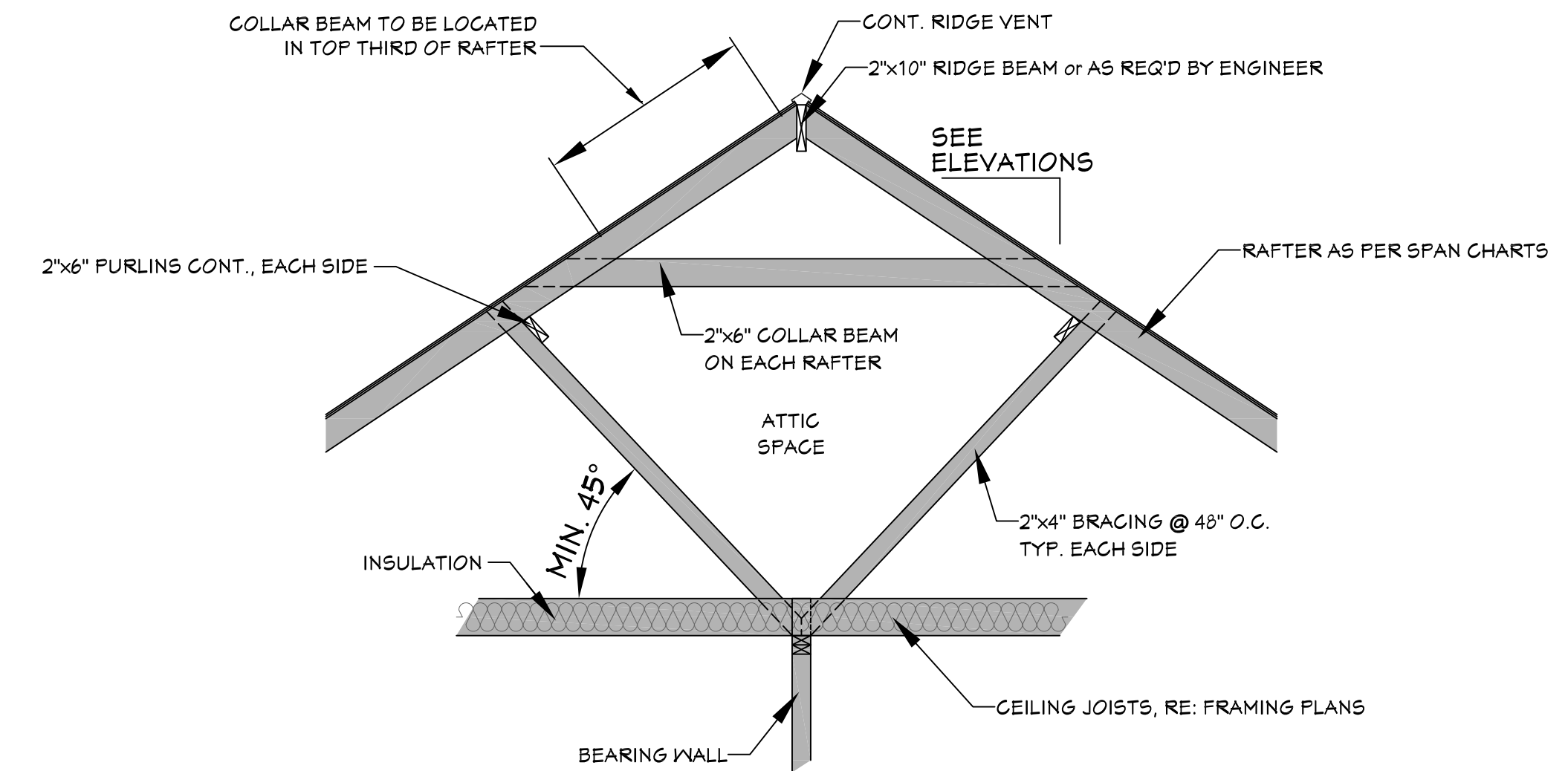
607 TYP. ROOF BRACING SCALE: N.T.S.
