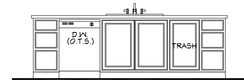
604 KITCHEN SCALE: 3/8" = 1'-0"
