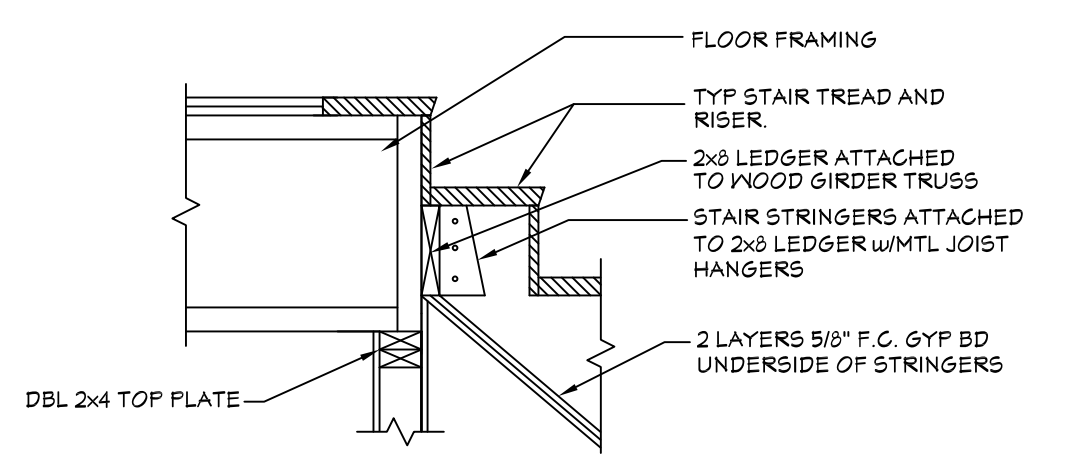
803 TYP. STAIR SECTION SCALE----- N.T.S.
