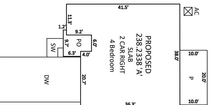
INSET SCALE: 1"=20'
