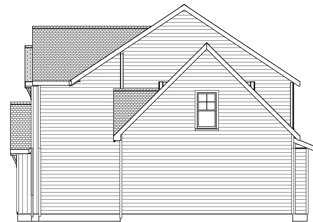
RIGHT ELEVATION
