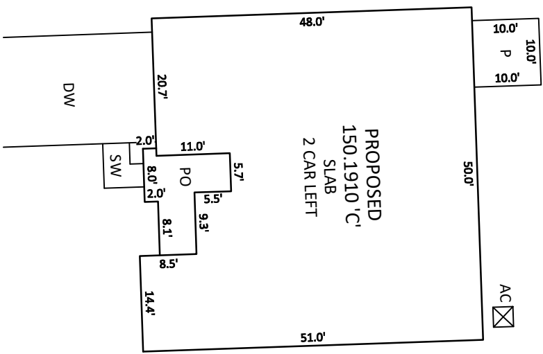
INSET SCALE: 1"=20'
