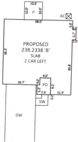
INSET SCALE: 1"=20'
