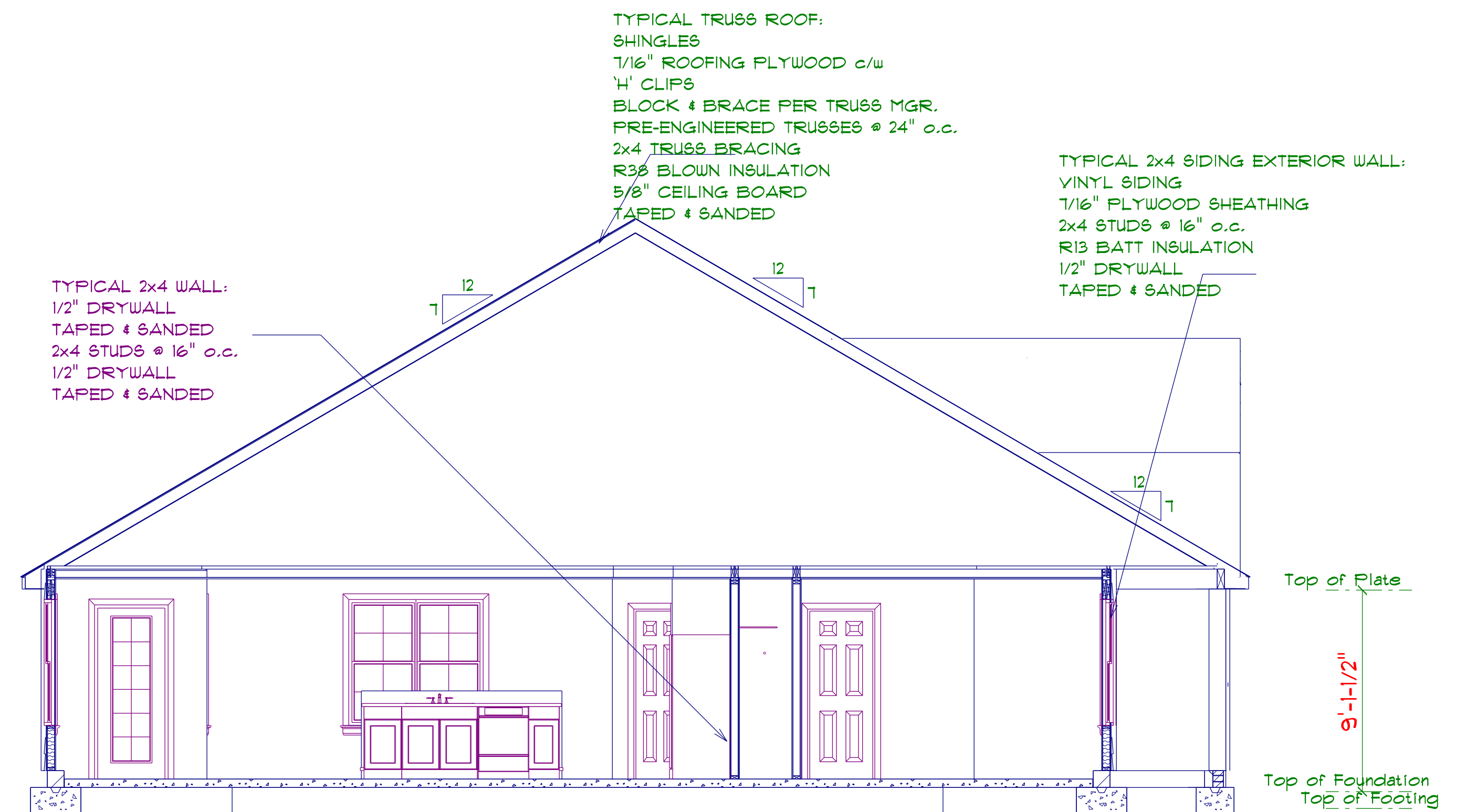
SECTION SCALE: 1" = 1/4"
