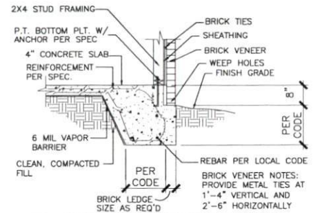
3 SECTION W/BRICK LEDGE N.T.S.
