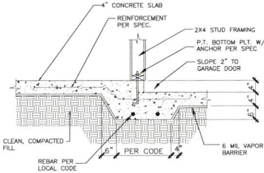
5 SECTION @ GARAGE N.T.S.
