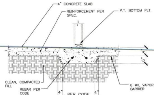
9 SECTION @ GRADE BEAM N.T.S.
