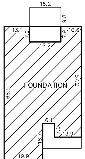
INSET N.T.S.
