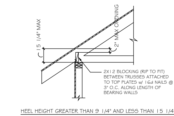
E TRUSS BLOCKING REQUIREMENTS N.T.S.
