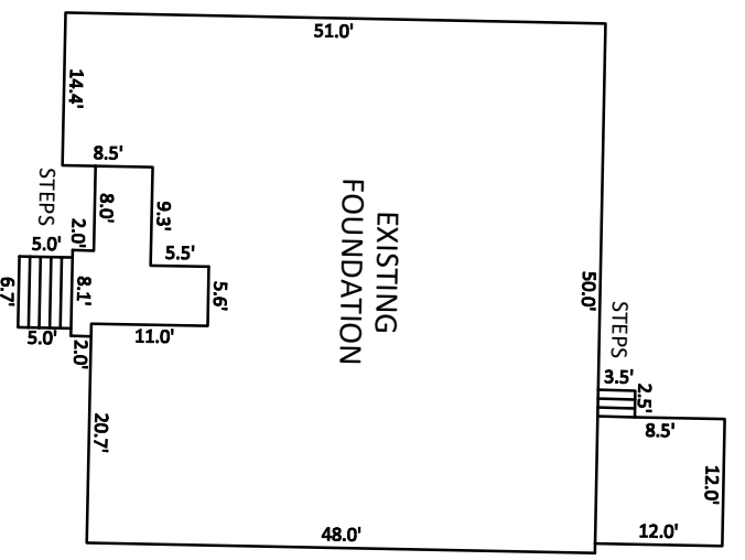
INSET SCALE: 1" = 20'
