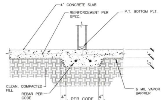
9 SECTION @ GRADE BEAM D1 N.T.S.
