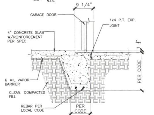
6 TYPICAL GARAGE DOOR DETAIL D1 N.T.S.
