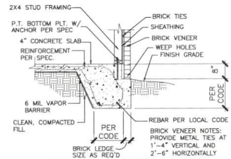
3 SECTION W/BRICK LEDGE D1 N.T.S.
