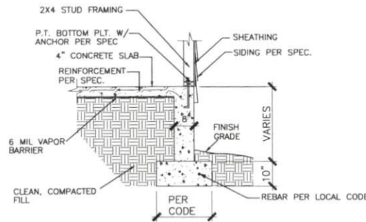
8 TYPICAL STEM WALL DETAIL D1 N.T.S.
