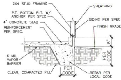
1 GARAGE CURB DETAIL D1 N.T.S.
