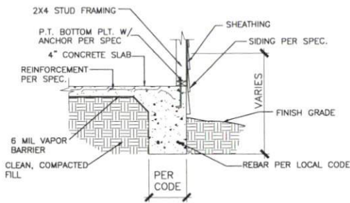
7 TYPICAL TURNDOWN SLAB DETAIL D1 N.T.S.
