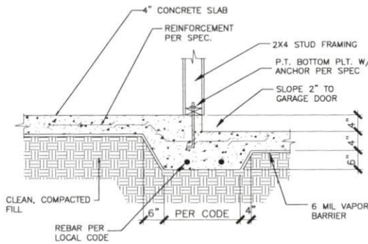
5 SECTION @ GARAGE D1 N.T.S.
