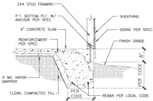
4 TYPICAL SLAB DETAIL D1 N.T.S.
