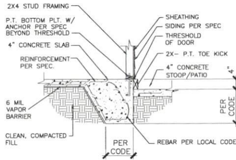
2 SECTION @ PORCH/PATIO D1 N.T.S.
