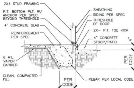
2 SECTION @ PORCH/PATIO N.T.S.
