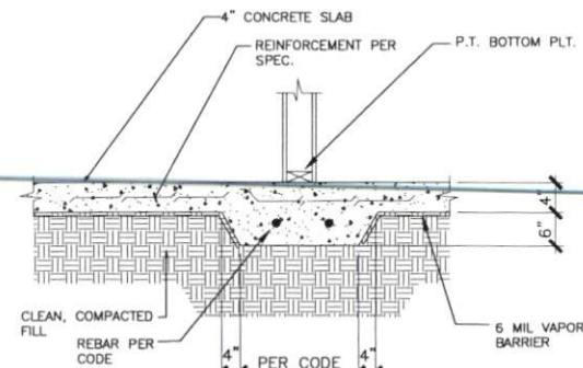
9 SECTION @ GRADE BEAM N.T.S.
