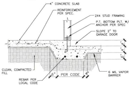
5 SECTION @ GARAGE N.T.S.
