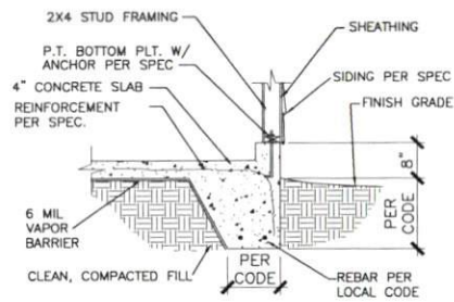
1 GARAGE CURB DETAIL N.T.S.
