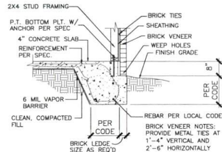
3 SECTION W/BRICK LEDGE N.T.S.
