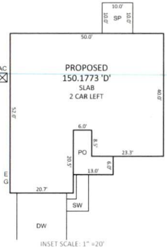
INSET SCALE: 1" = 20'
