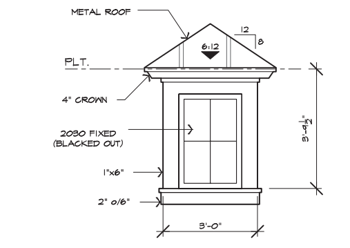
TYP. HIP DORMER
