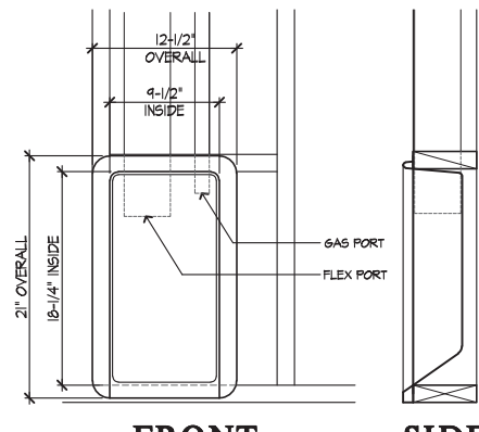
FRONT SIDE DRYER BOX DETAIL 149 SCALE: N.T.S. ADB-149 ADB
