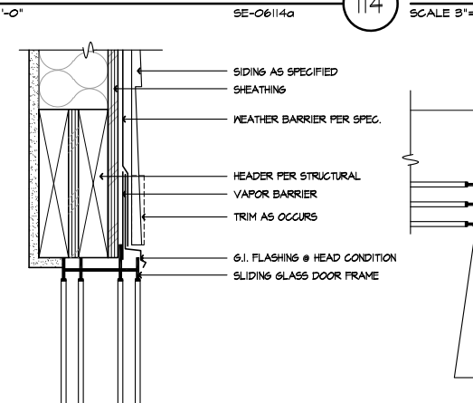
115 SLDG. DOOR HEAD-SIDING SCALE 3"=1'-0" SE-06115a
