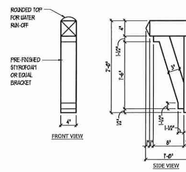
BRACKET DETAIL SCALE: 1" = 1'-0"
