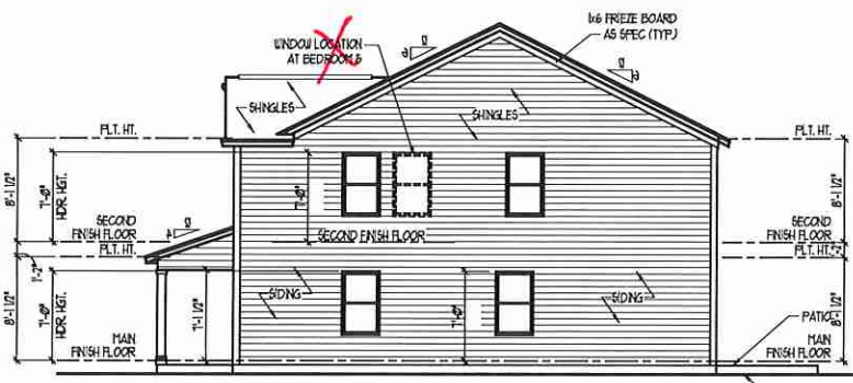
RIGHT ELEVATION
