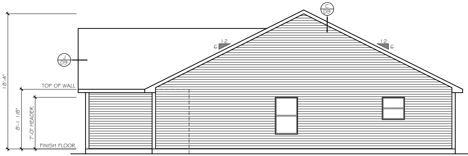
RIGHT ELEVATION
