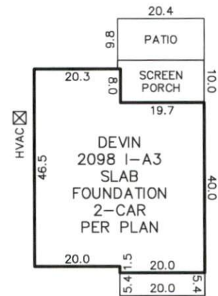
INSET N.T.S.
