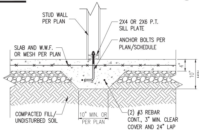
D1s 3/4" = 1'-0"
