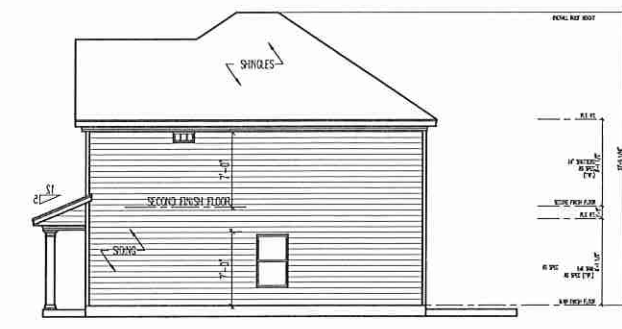
RIGHT ELEVATION SCALE: 1/8" = 1'-0"
