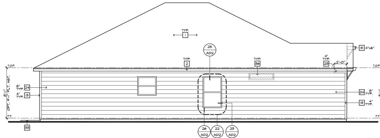
LEFT ELEVATION 'B'
