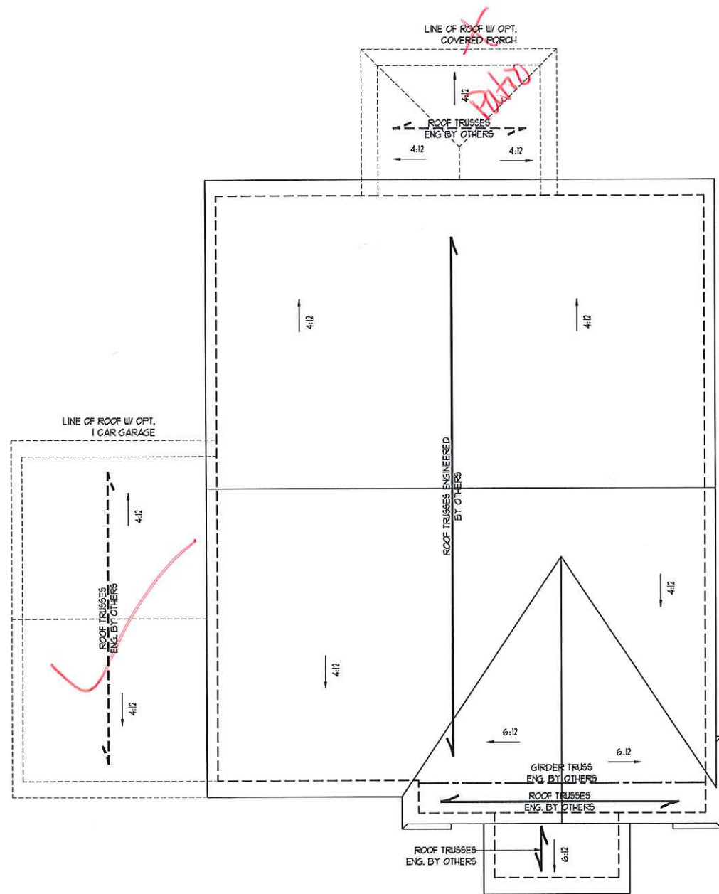
ELEVATION A
