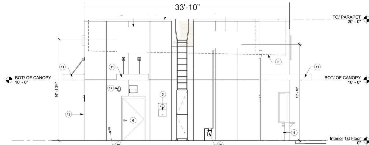
2 EAST ELEVATION Scale: 1/8" = 1'-0"
