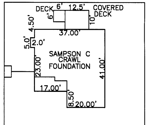
INSET, SCALE: 1"=30'
