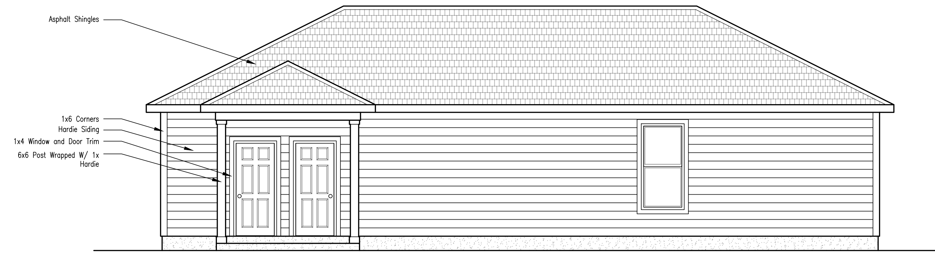
Right Elevation
