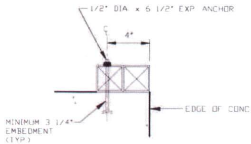
SECTION 1 SCALE: NTS
