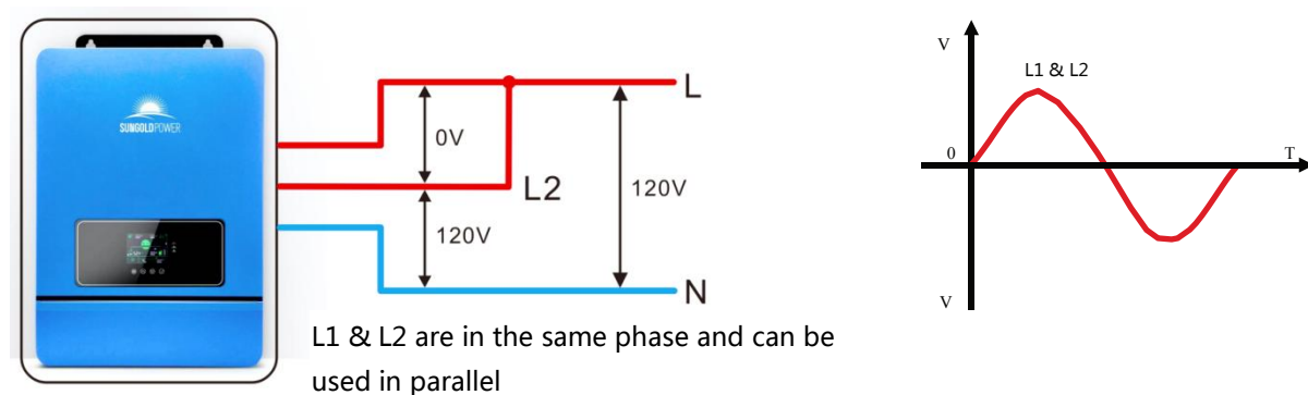
AC output
