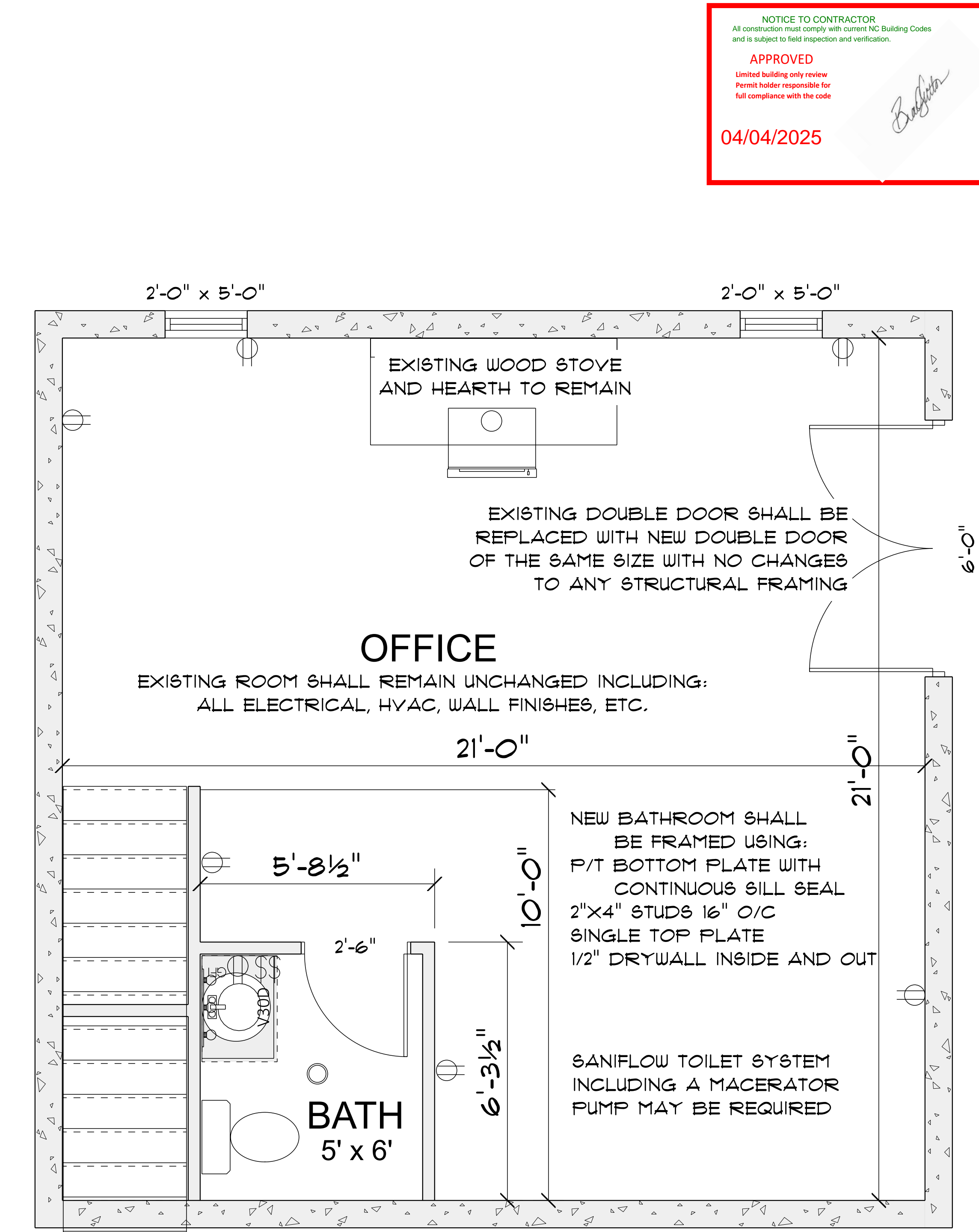
LAYOUT SCALE: 1/2" = 1'-0"
