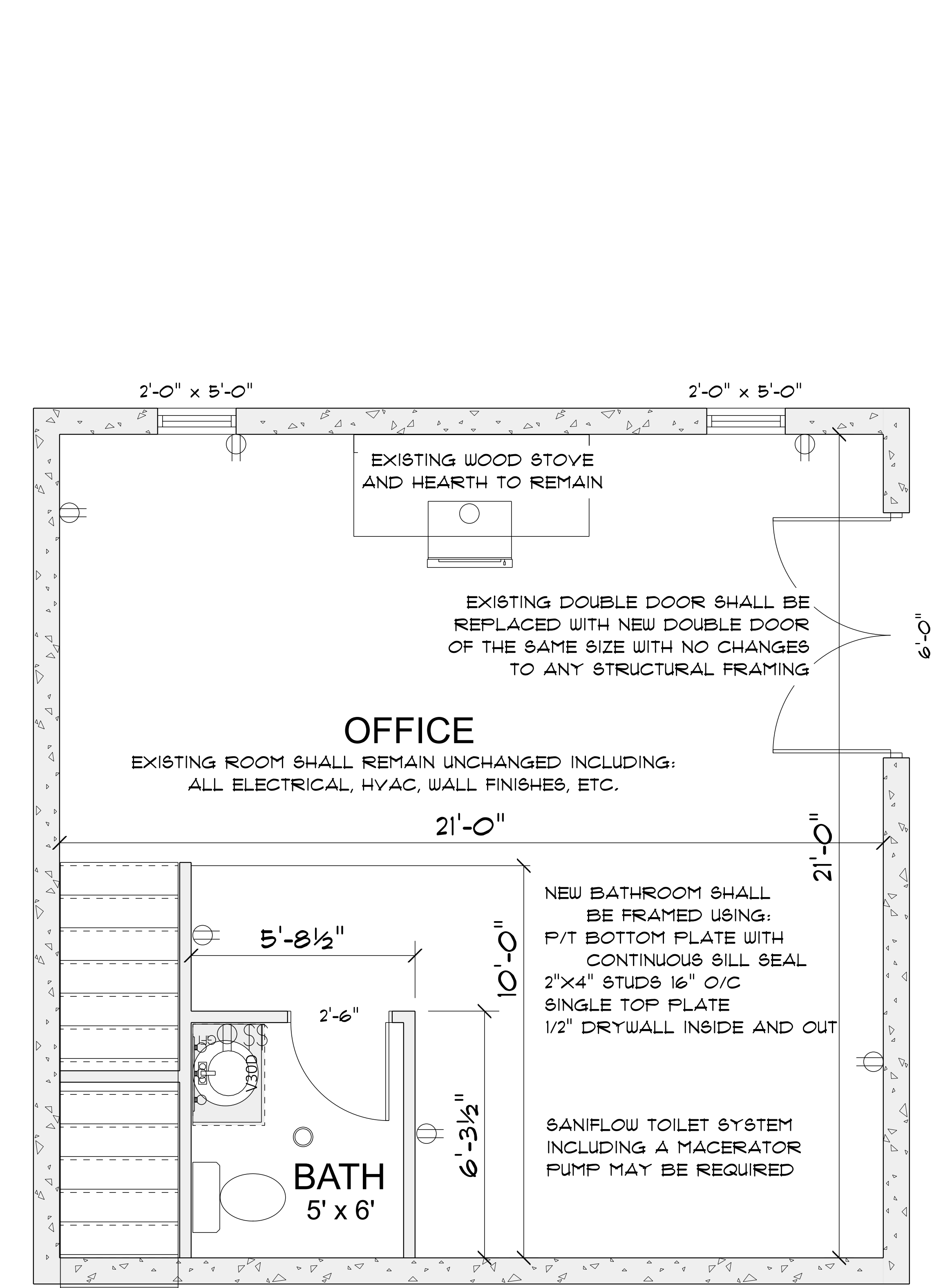
LAYOUT SCALE: 1/2" = 1'-0"
