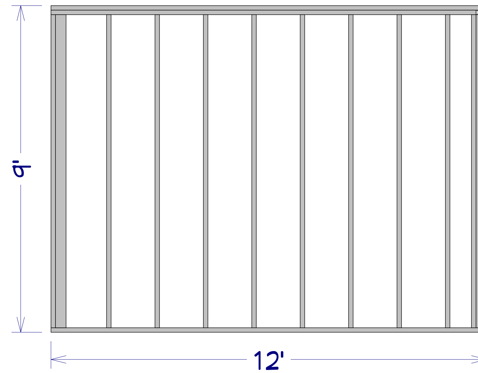
E3 - WALL FRAMING
