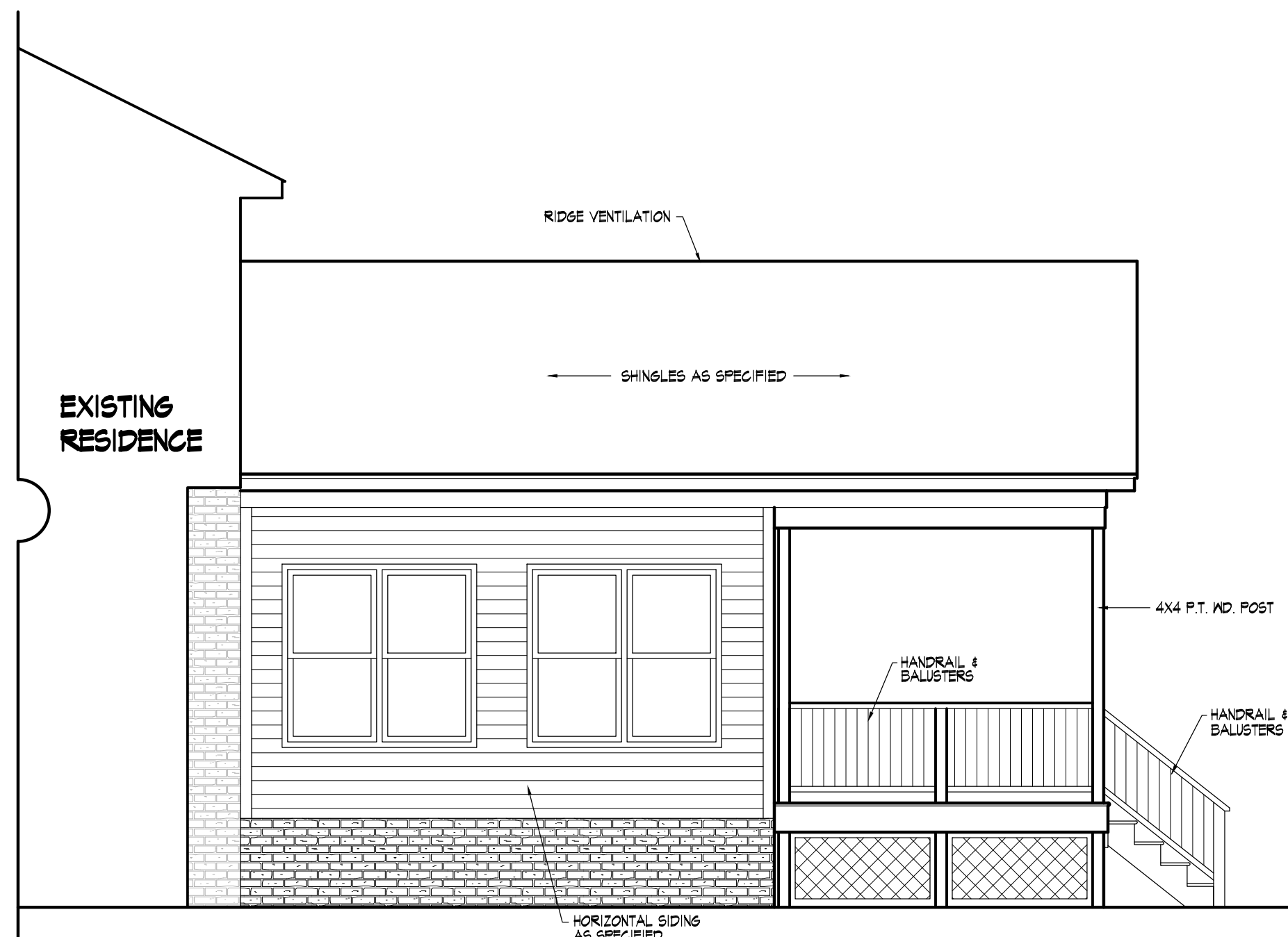
203 Right Elevation
