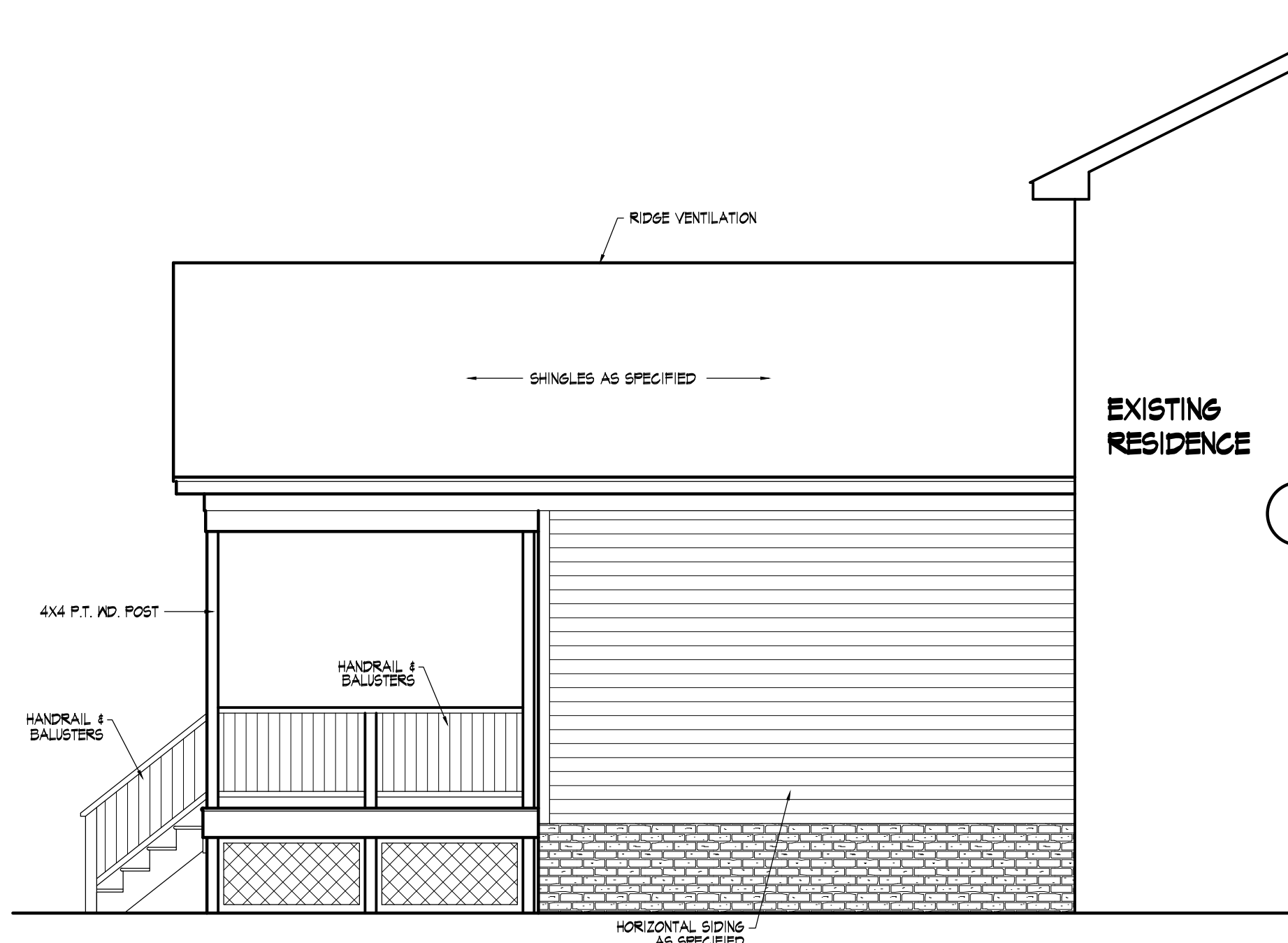
202 Left Elevation
